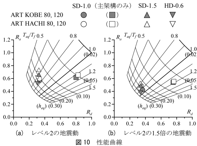
図 10 性能曲線
